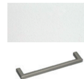
Garderoben | Einbauschränke Fronten Kunstharz, weiss belegt Kanten ABS 0.8mm, umlaufend Bügelgriff, Edelstahl Garderobenteil mit Kleiderstange und Tablare, Putzschrank
